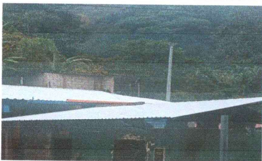
Foto 5: Proceso de ejecución de instalación de lámina troquelada calibre 26 en el módulo de la cocina.
