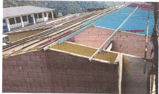
Foto 2: Vista desde otro angulo la desmantelación de láminas de zinc para su sustitución por lámina troquelada calibre 26 en módulo 1.
