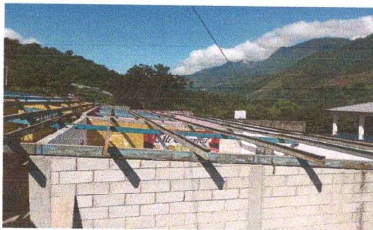
Foto 3: Trabajo de cubierta de lámina con la desmantelación de existentes para ser remplazadas con lámina troquelada calibre 26 en el módulo 2.
